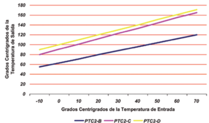
Temperatura de entrada vs. salida de la resistencia
